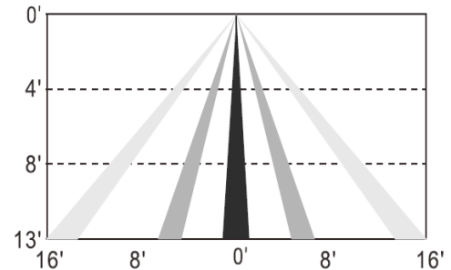
Couverture des détecteurs de mouvement à micro-ondes
